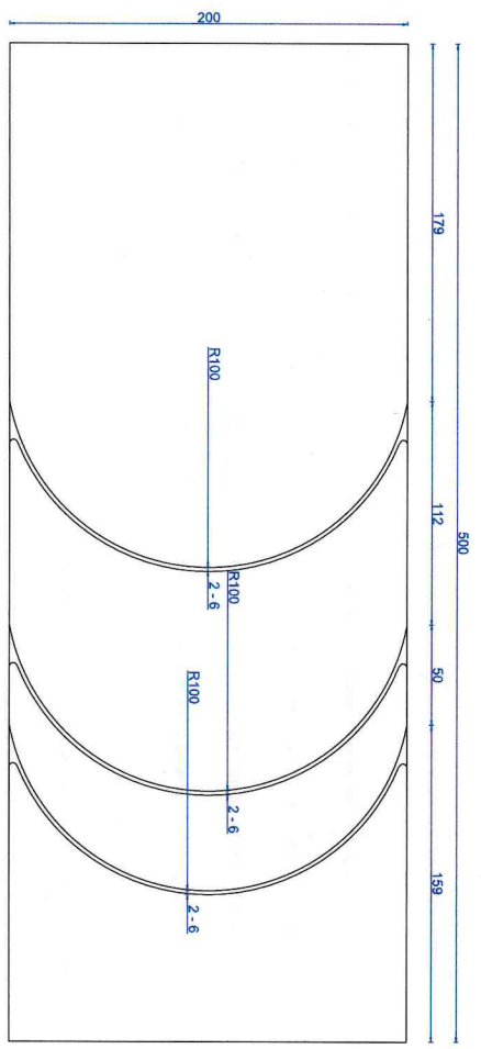
pôdorys
