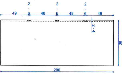
priečny rez
