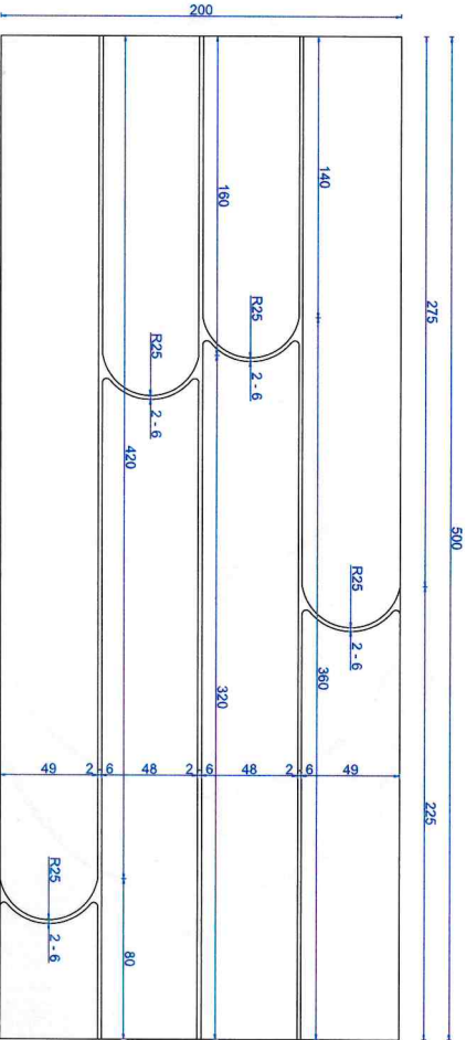
pôdorys
